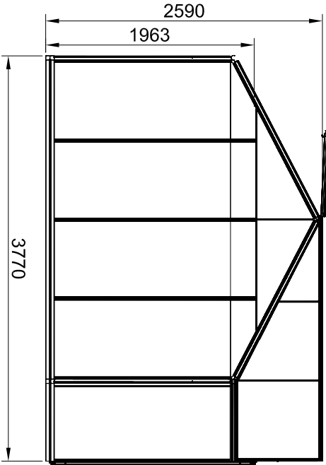
Right/leftview
